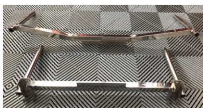
“Heavy Duty” Tube, ojačana cijevna krma
